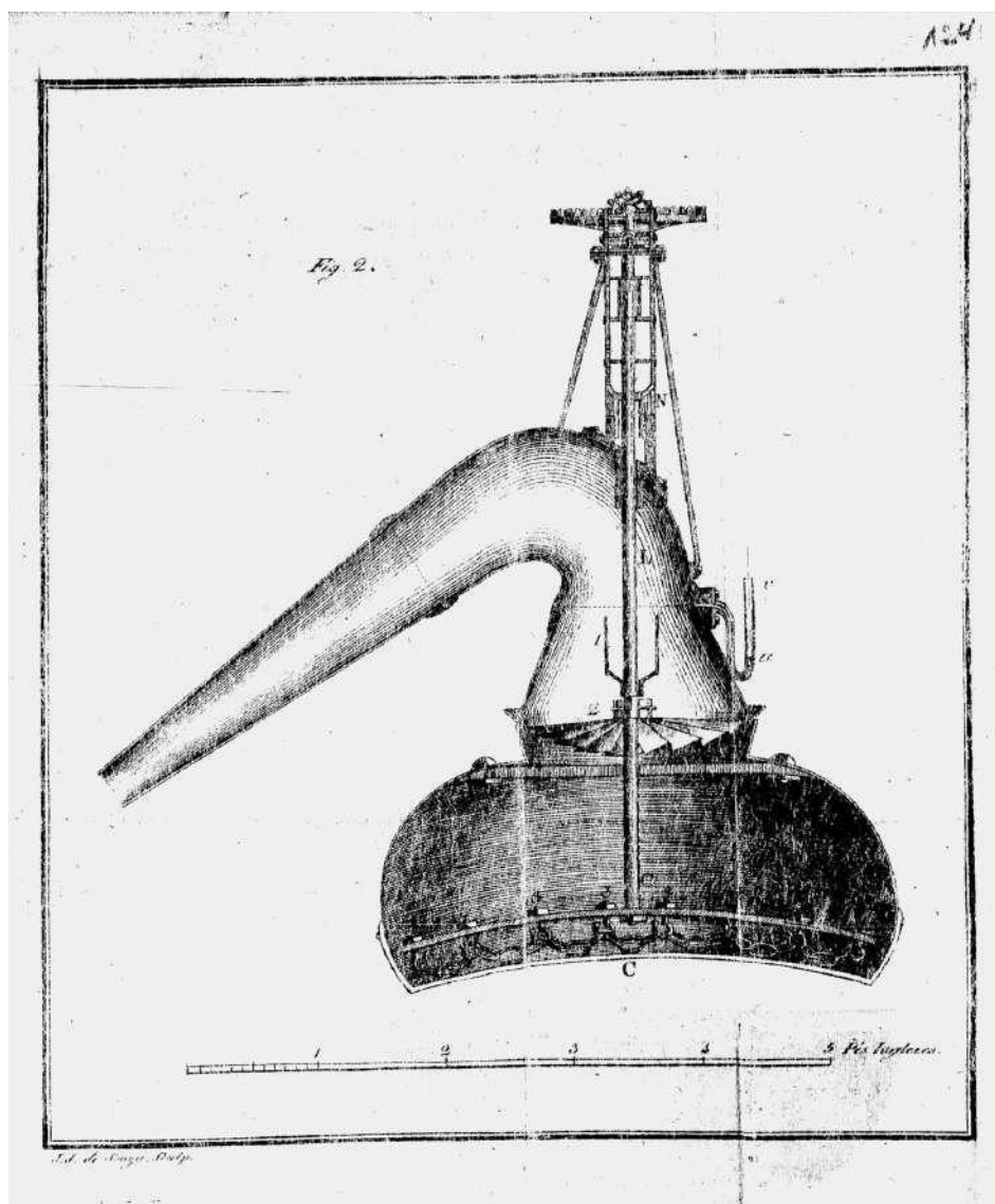
Fig.41 - Reprodução do alambique descrito por Gaspar Mendes em seu artigo no jornal O Patriota , em 1813. 2ª edição, página 115.
